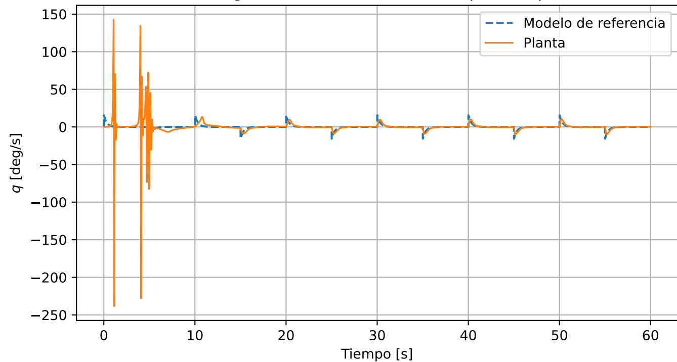
Seguimiento MRAC con tren de pulsos: q
